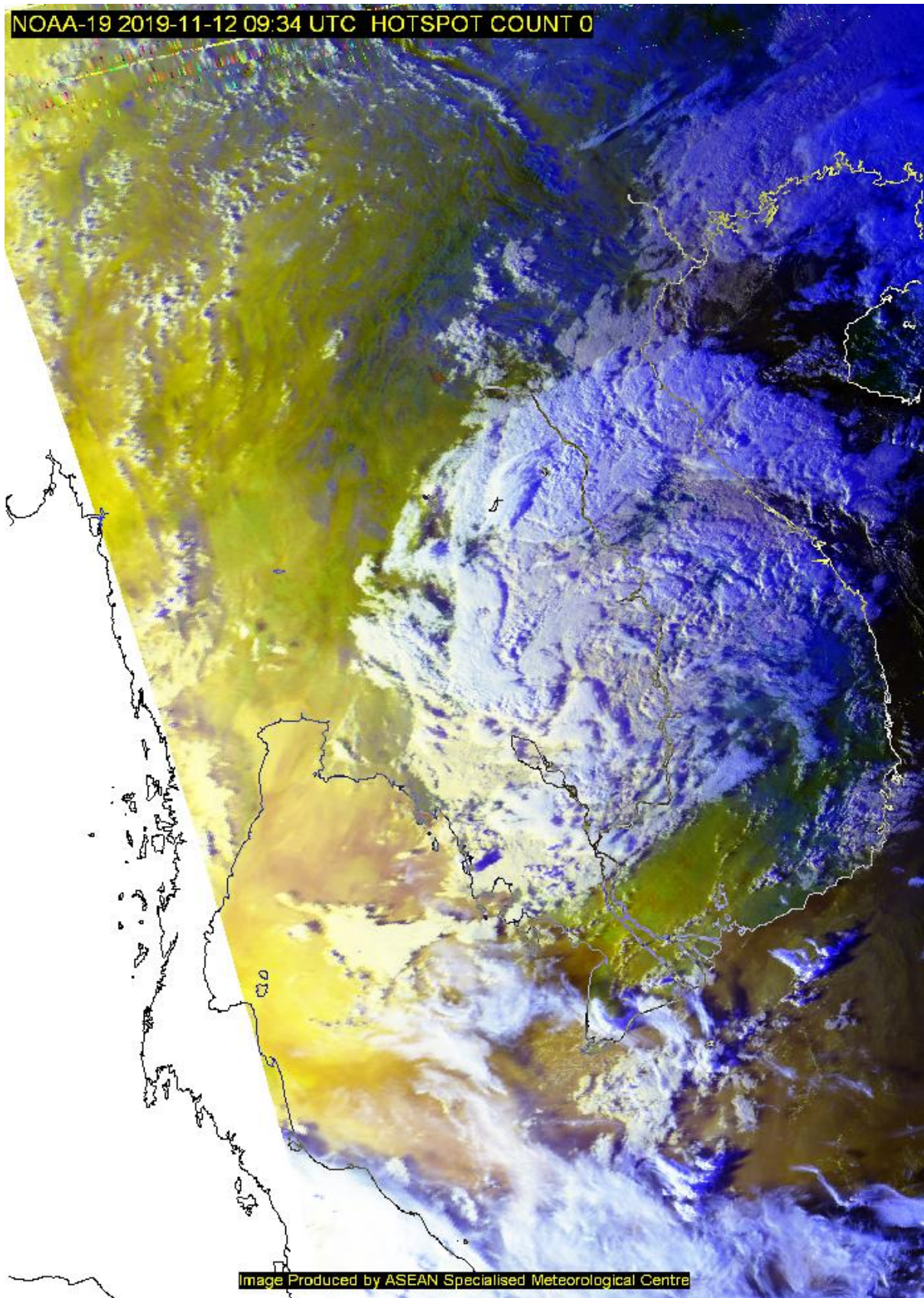
รูปที่ 1 แสดงจำนวนและตำแหน่งจุด Hotspot โชนอินโดจีน ซึ่งแปลผลจากภาพถ่ายดาวเทียม NOAA-19 วันที่ 12 พฤศจิกายน 2562
